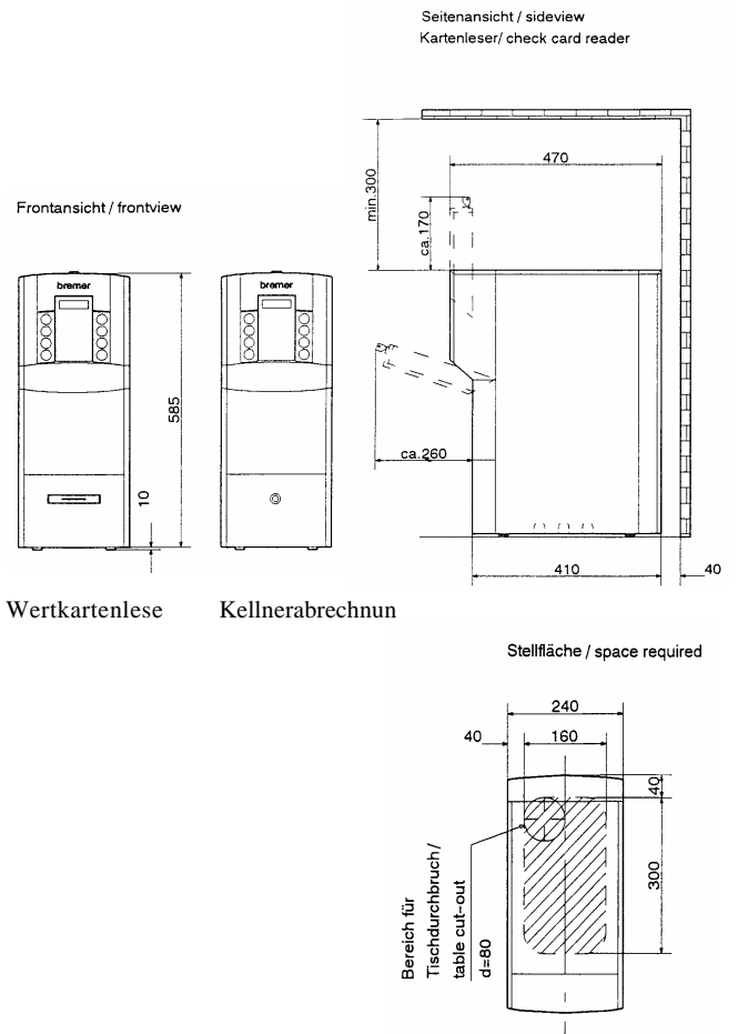
Tischedurchbruch d=80 innerhalb der schraffierten
